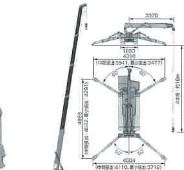
2.98t吊かにクレーン
