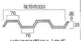
YSY35W型アルミ矢板
