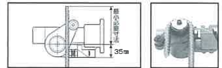
16mmポータブルバンダー
